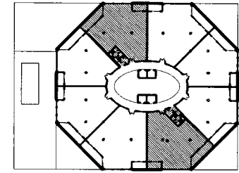
KEY PLAN - LEVELS 7-16 N.T.S.
